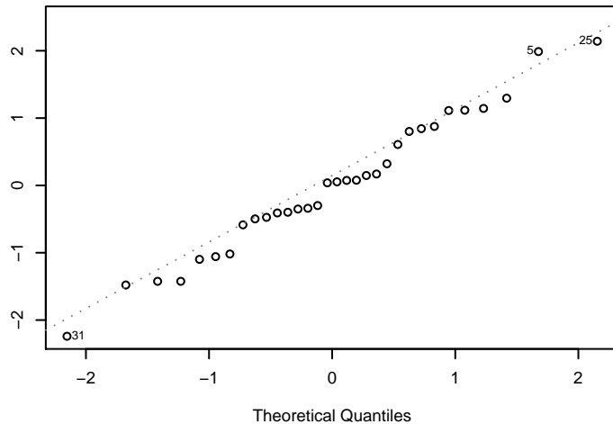
Normal Q-Q
